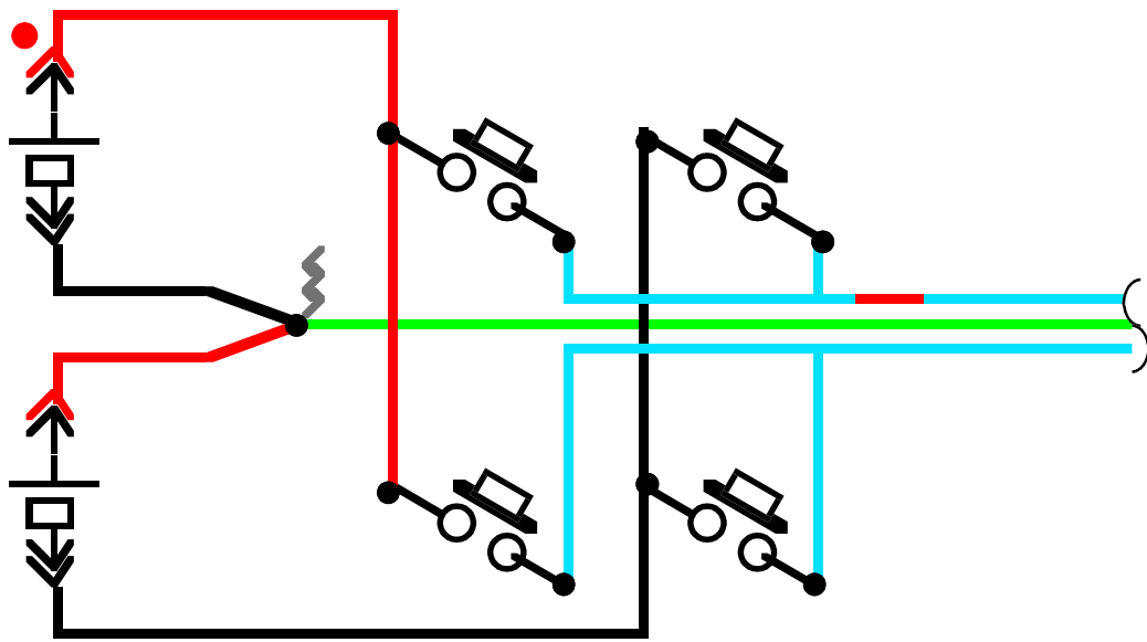
コントローラ部回路
