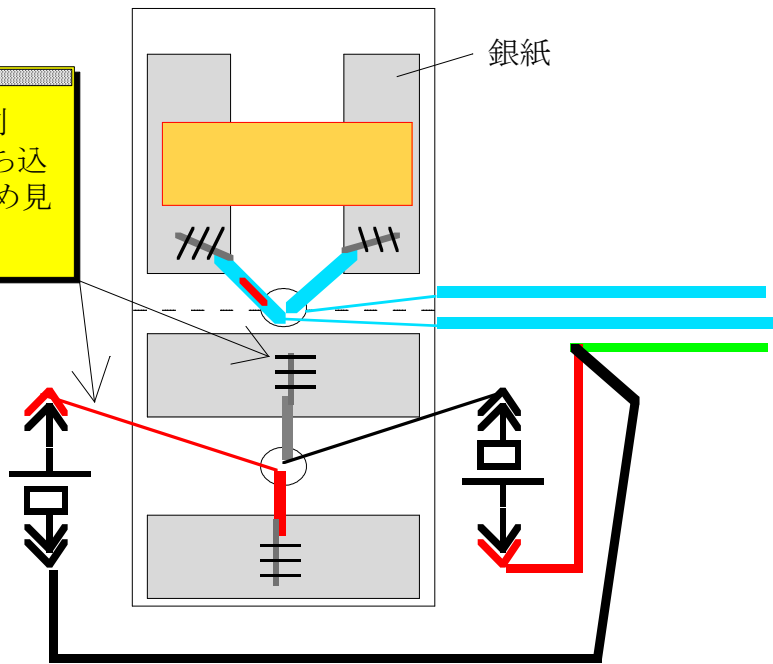
コントローラ部実態配線
